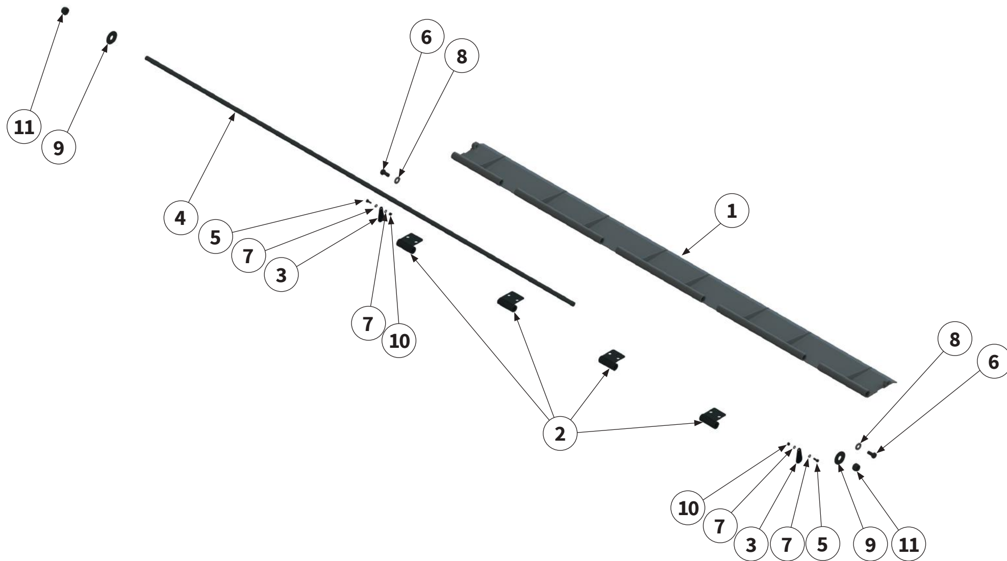
KURZSCHNITTKLAPPE | Short-cut flap | Clapet de coupe courte | Tapa de corte corto |
